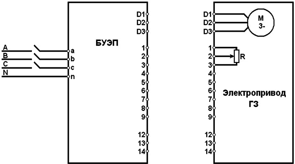
Рис.5 (1) Блок-схема подключения БУЭП к электроприводу (для электросхемы на рис.4 (1))
