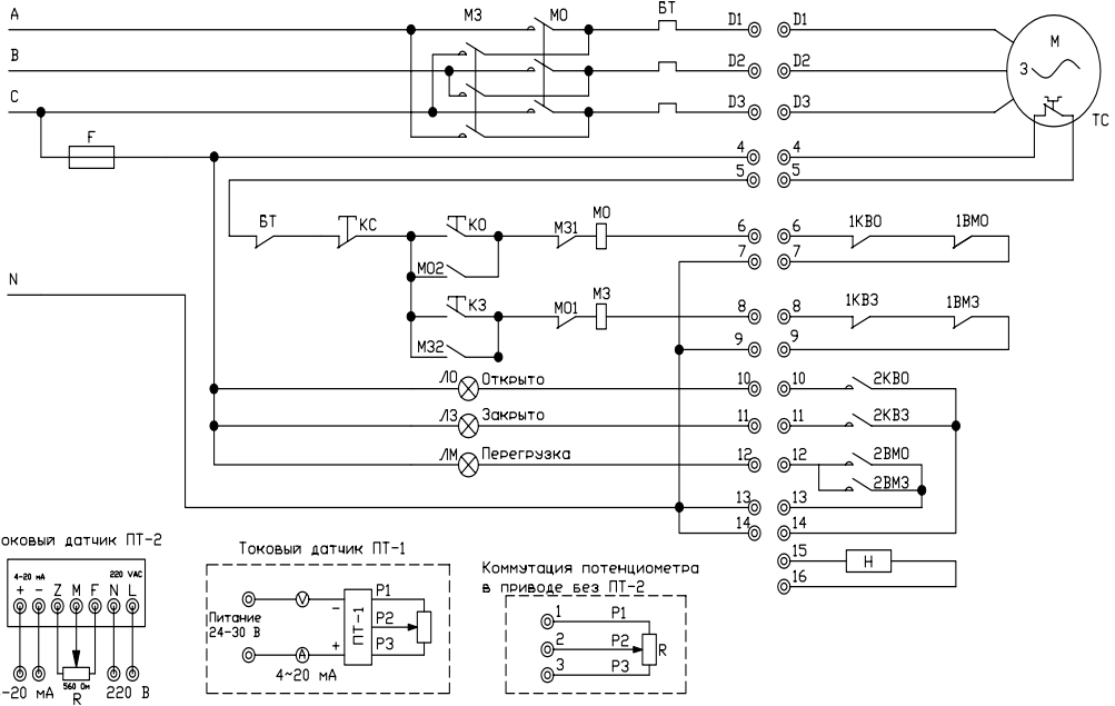
Рис.4 (2) Электрическая схема управления (обновленная схема)
