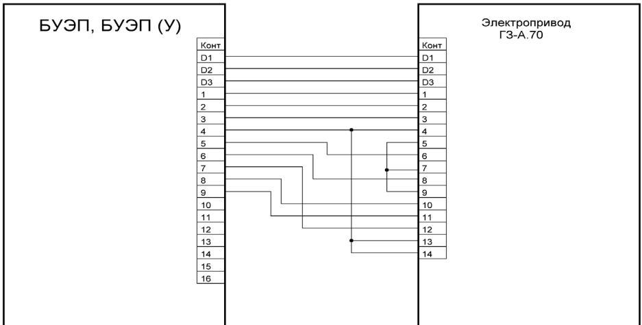
Рис.5 (1) Блок-схема подключения БУЭП к электроприводу (для электросхемы на рис.4 (1))
