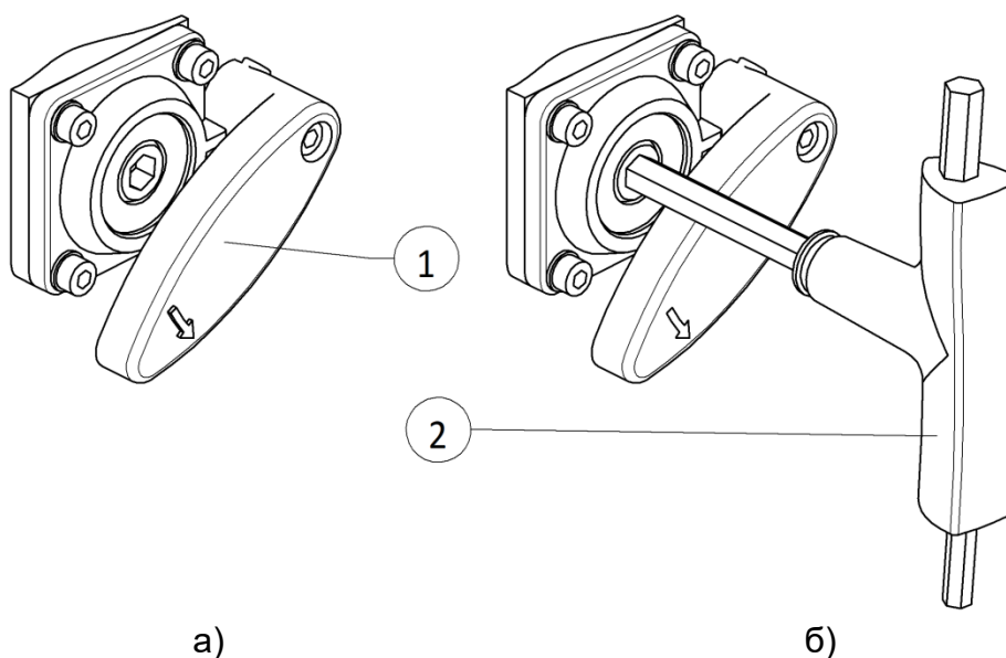
Рисунок 6 – Переключение на ручное управление 1 – Рычаг переключения режимов, 2 – Рукоятка.
