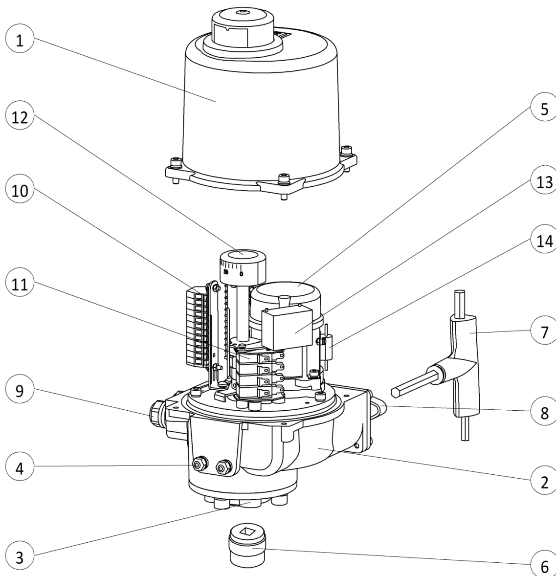
Рисунок 1 – Общий вид электропривода
