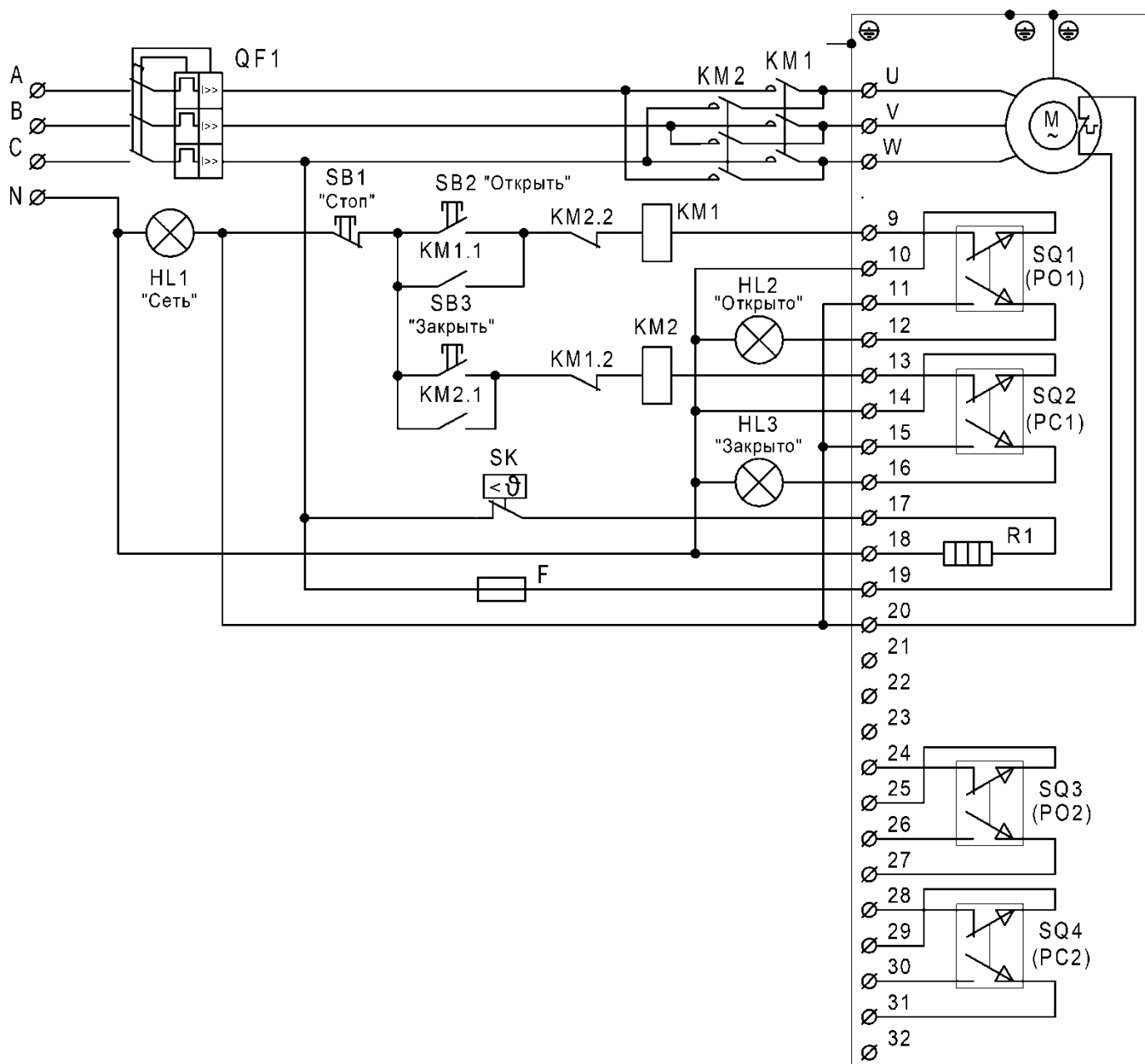
Рисунок Б.2 – Схема подключения электропривода с трехфазным электродвигателем
