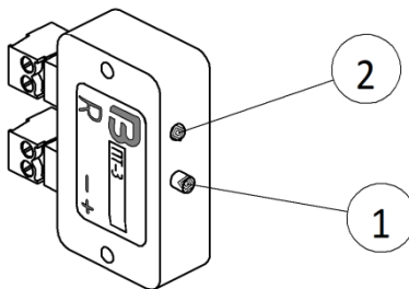
Рисунок 14 – Токовый датчик ПТЗ 1 – Кнопка, 2 – Светодиодный индикатор.
