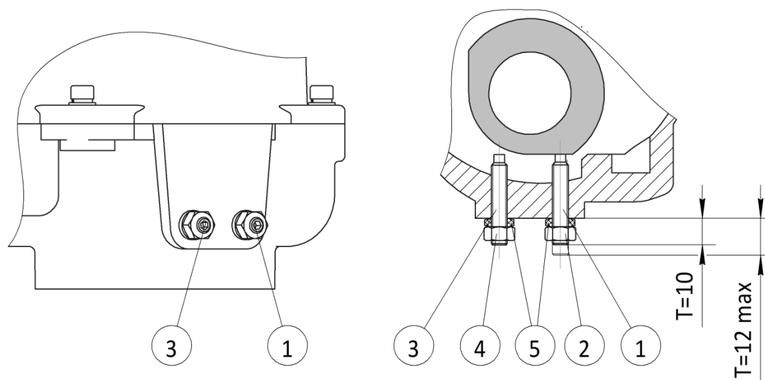
Рисунок 7 – Концевые упоры
