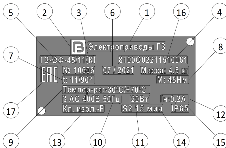
Рисунок 2 – Заводская табличка электропривода (пример)
