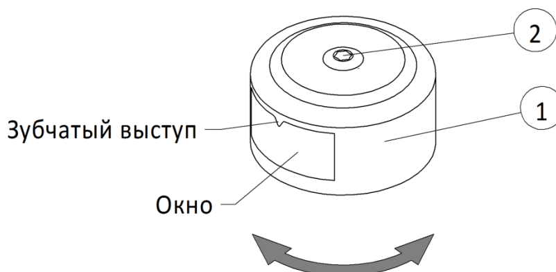
Рисунок 11 – Регулировка положения окна указателя 1 – Крышка указателя, 2 – Винт
