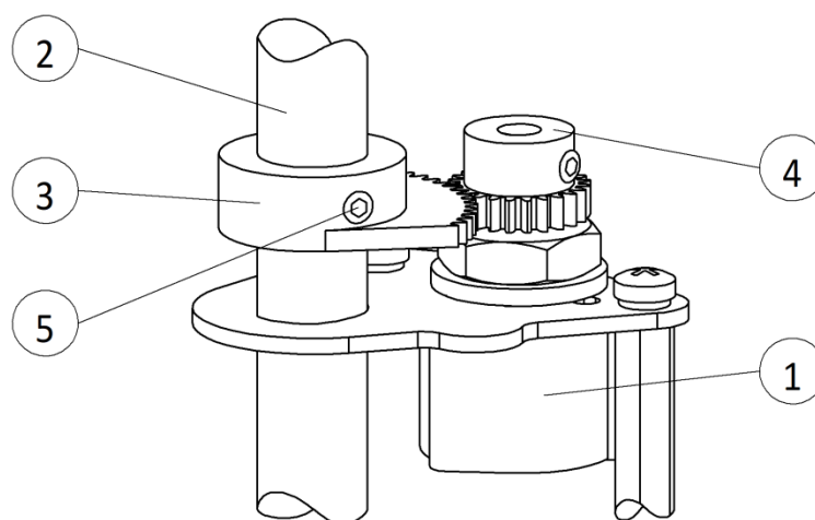
Рисунок 13 – Датчик омический 1 – Потенциометр, 2 – Вал указателя, 3 – Зубчатый сектор, 4 – Шестерня, 5 – Винт установочный
