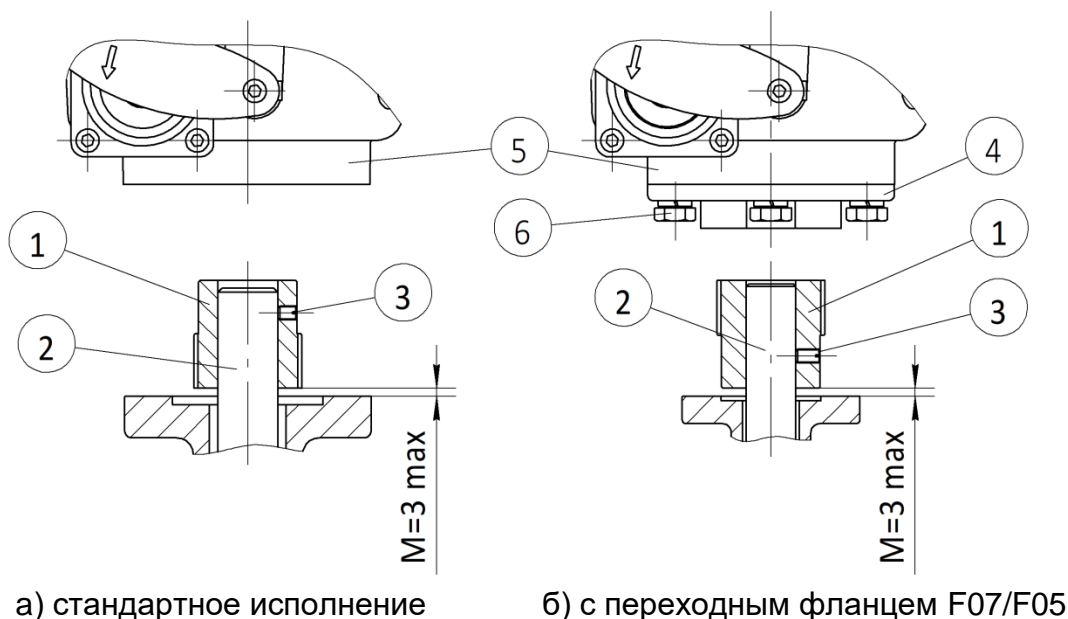
Рисунок 4 – Установка соединительной втулки
