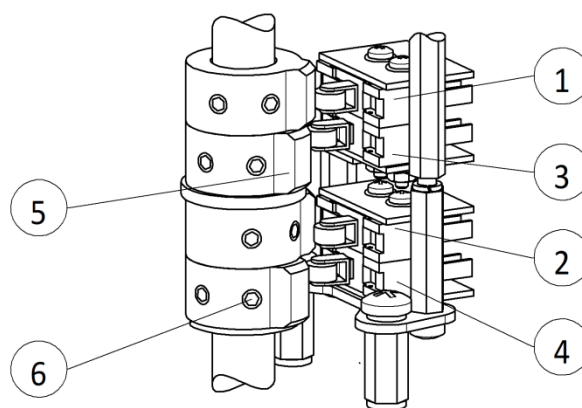
Рисунок 8 – Ограничитель хода с выключателями
