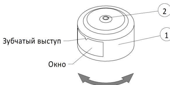
Рисунок 13 – Регулировка положения окна указателя 1 – Крышка указателя, 2 – Винт
