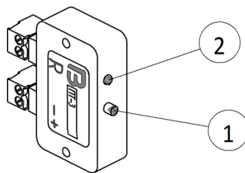
Рисунок 16 – Токвый датчик ПТЗ
