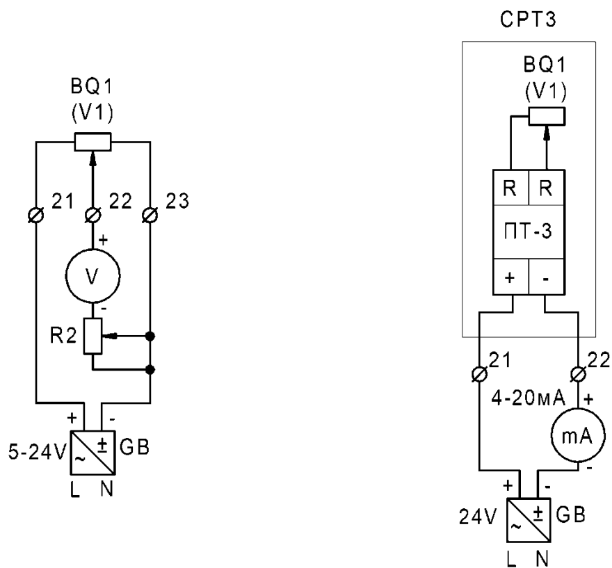
Рисунок Б.2 – Схемы подключения дополнительного оснащения привода (опции)
