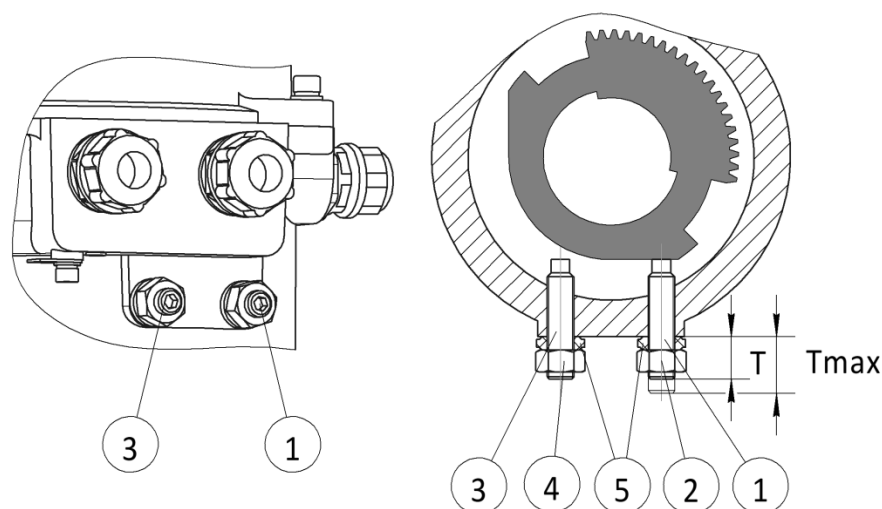
Рисунок 8 – Концевые упоры
