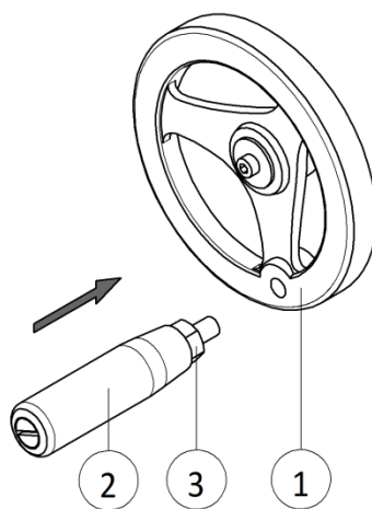
Рисунок 3 – Установка рукоятки
