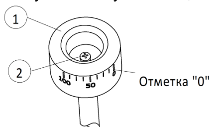
Рисунок 14 – Регулировка указателя положения 1 – Лимб, 2 – Винт
