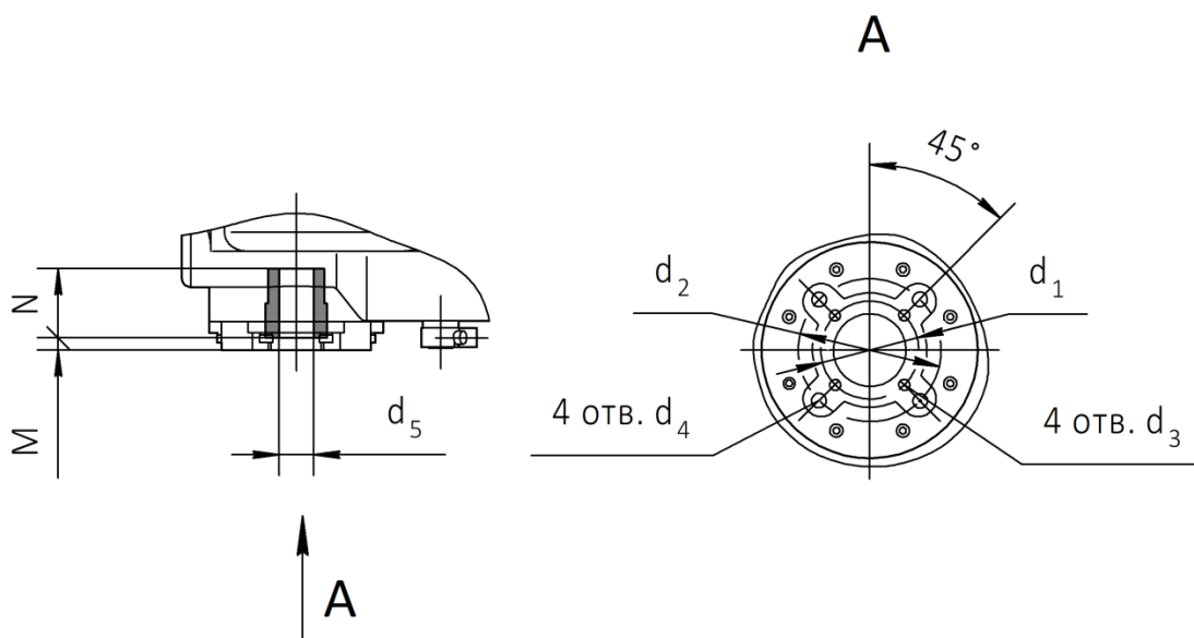
Рисунок А.2 – Присоединительные размеры электропривода
