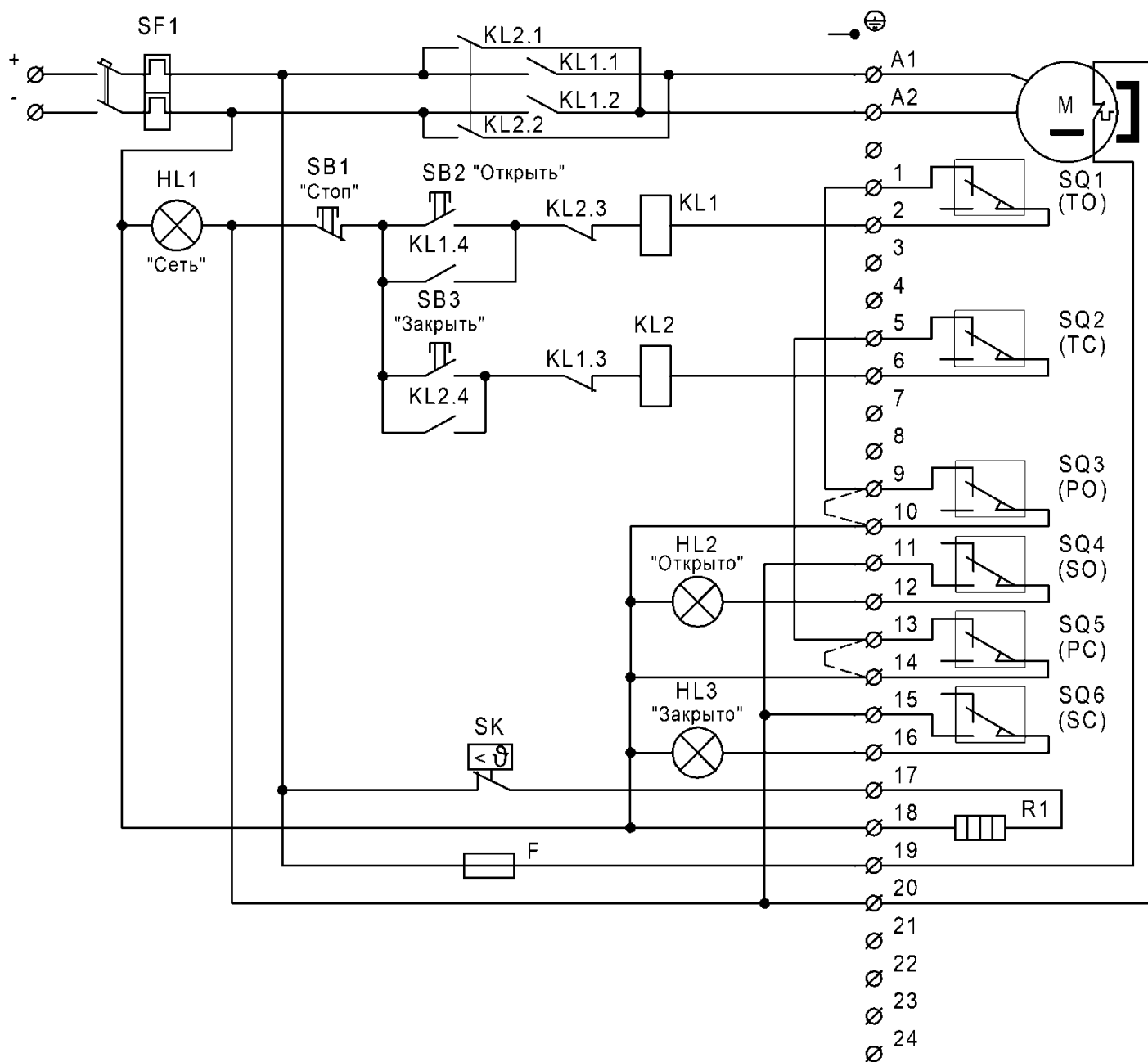
Рисунок Б.1 – Схема подключения электропривода
