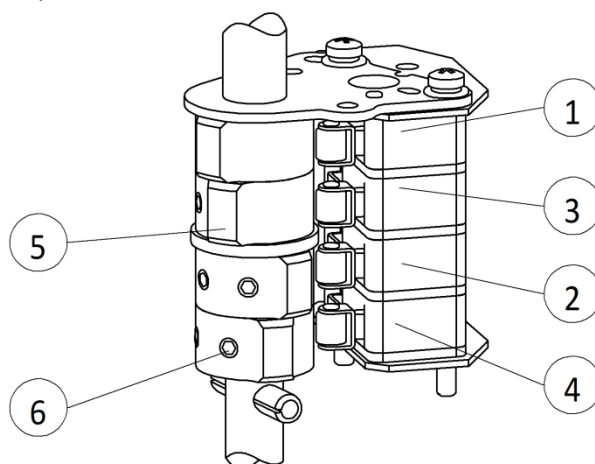
Рисунок 10 – Ограничитель хода с концевыми выключателями
